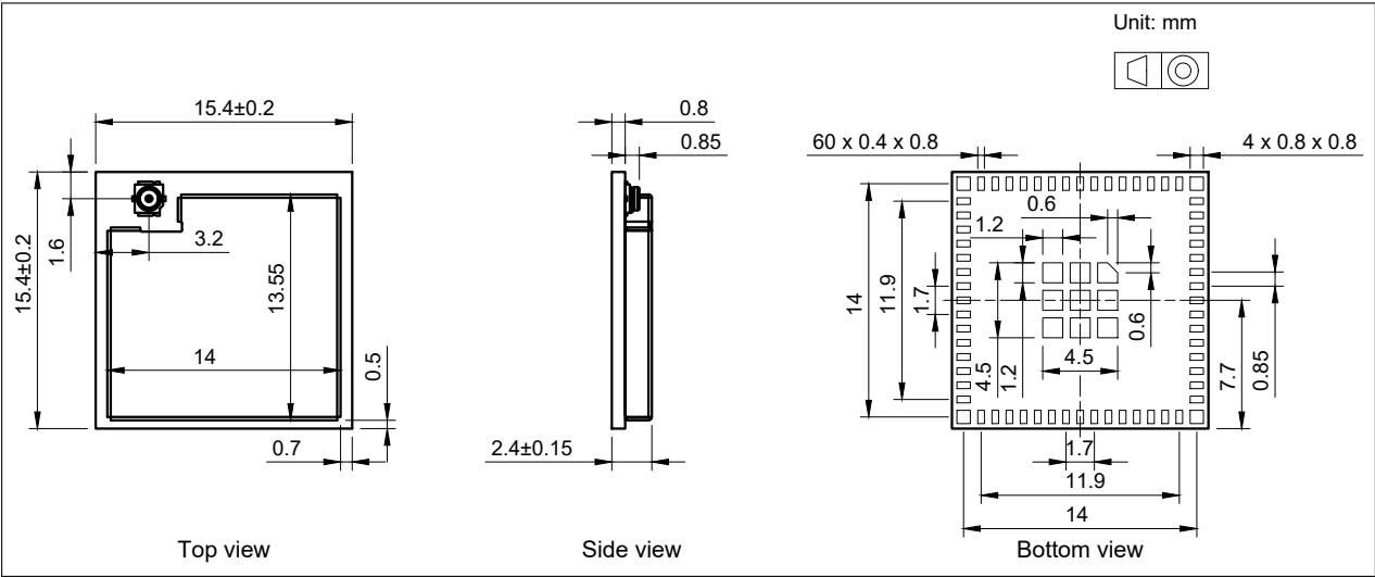
图 10-2. ESP32-S3-MINI-1U 模组尺寸
