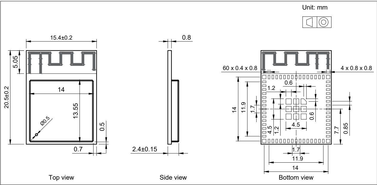
图 10-1. ESP32-S3-MINI-1 模组尺寸
