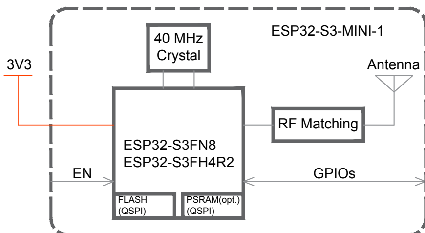
图 2-1. ESP32-S3-MINI-1 功能框图
