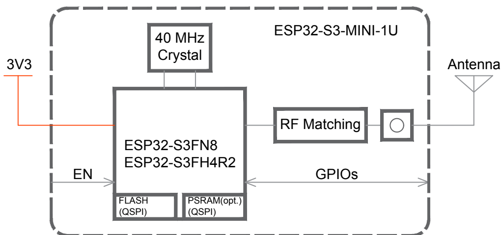
图 2-2. ESP32-S3-MINI-1U 功能框图
