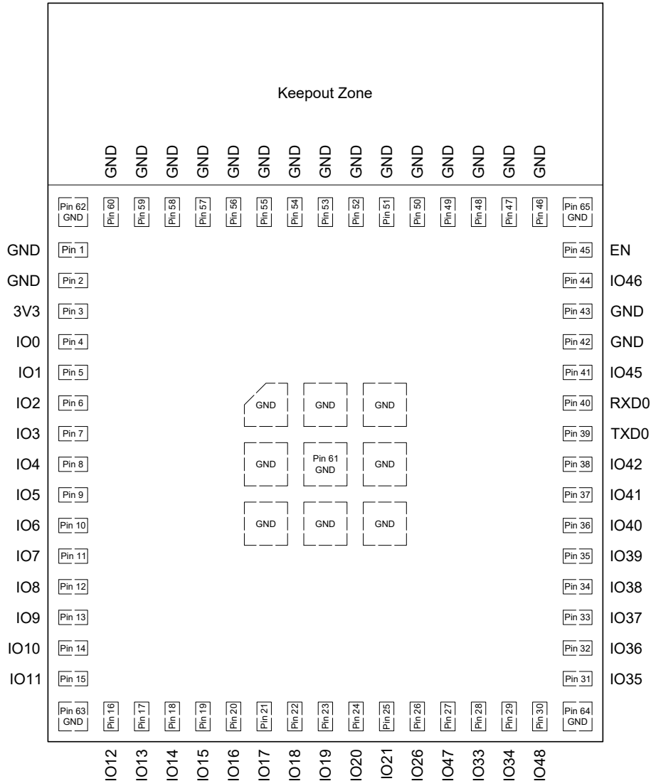
图 3-1. 管脚布局（顶视图）
