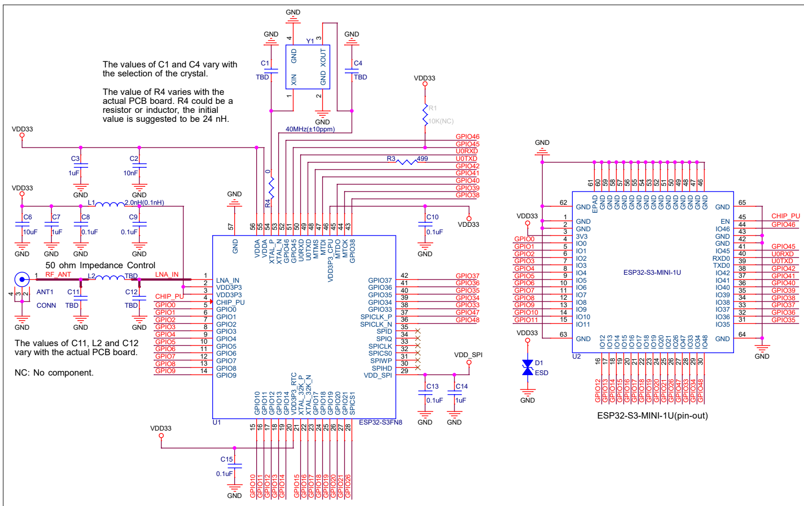
图 8-2. ESP32-S3-MINI-1U 原理图
