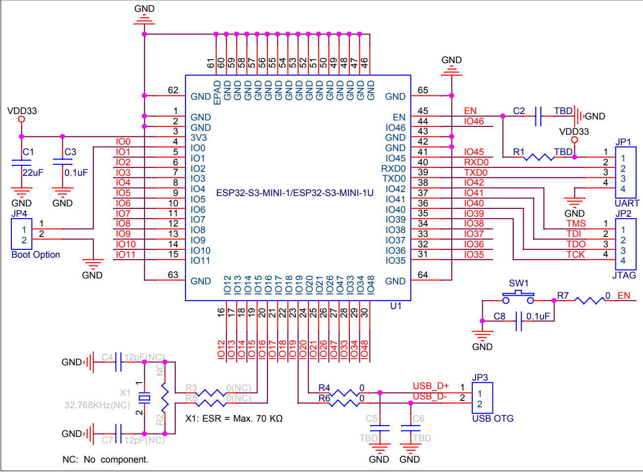
图 9-1. 外围设计原理图
