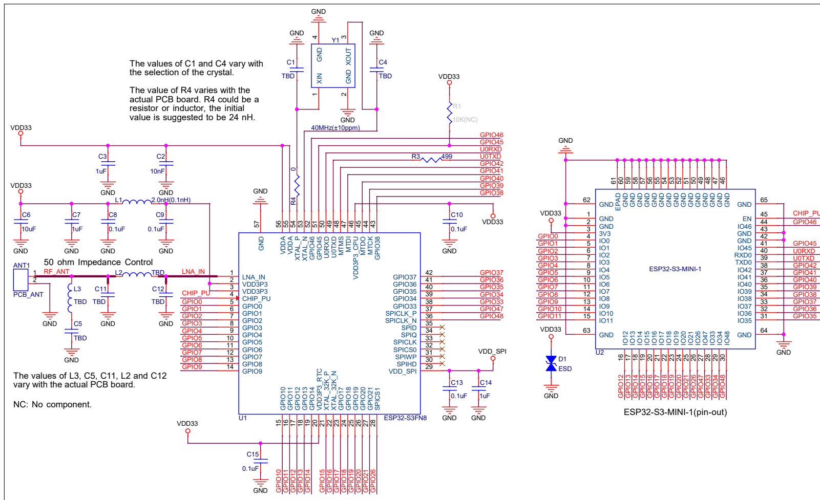
图 8-1. ESP32-S3-MINI-1 原理图
