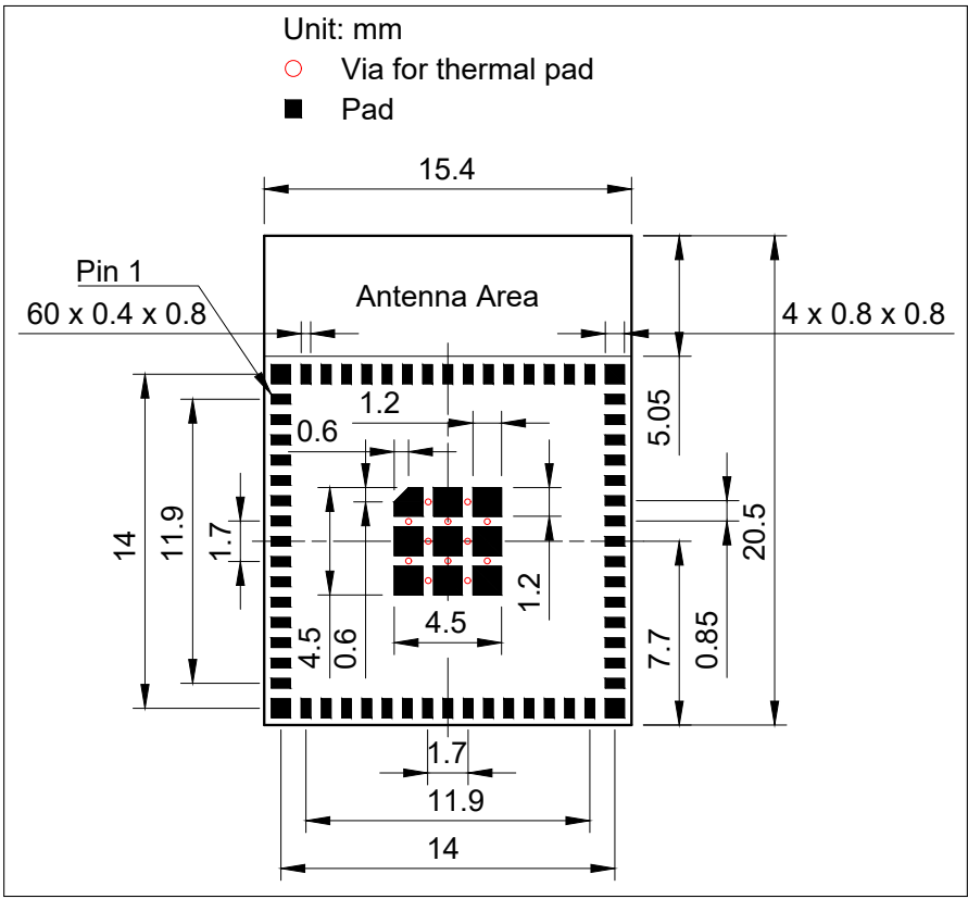
图 11-1. ESP32-S3-MINI-1 推荐 PCB 封装图
