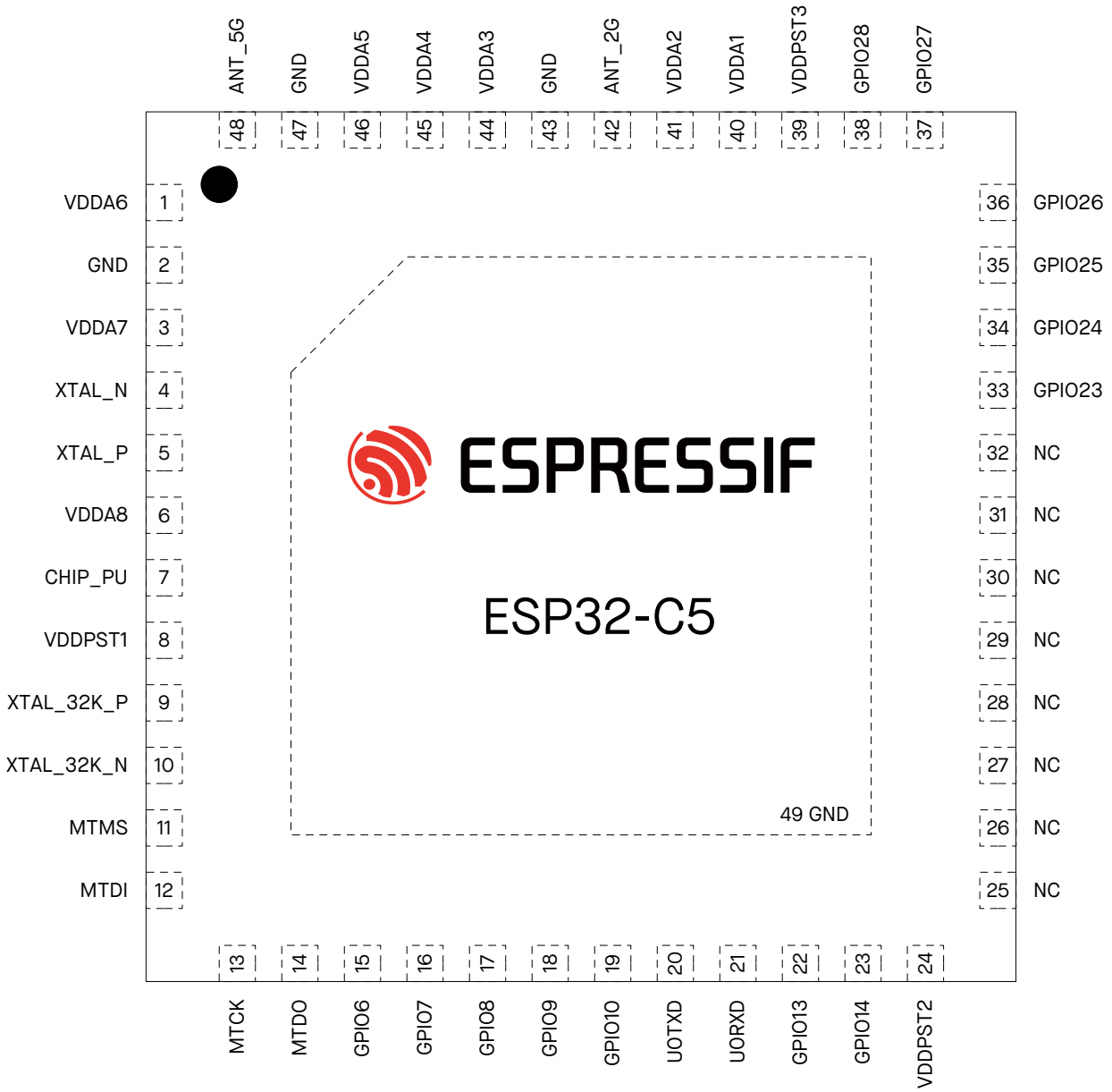
图 2-3. ESP32-C5NF8R2LA 管脚布局（俯视图）
