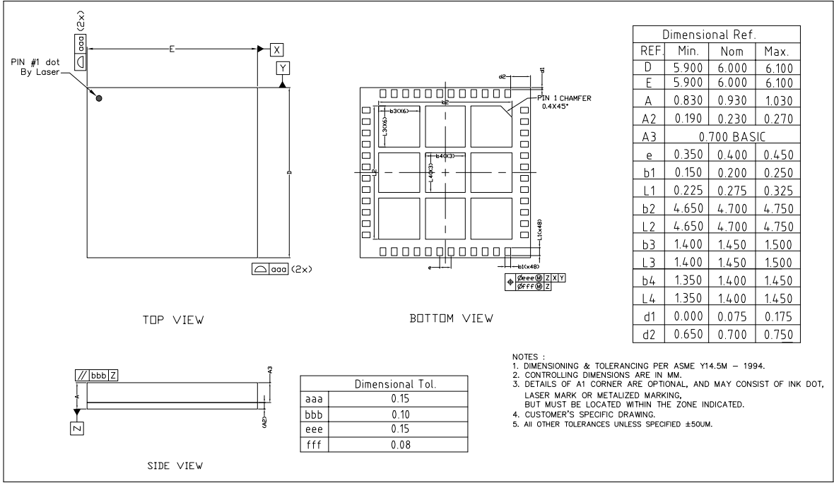
图 7-2. LGA48 (6 × 6 mm) 封装
