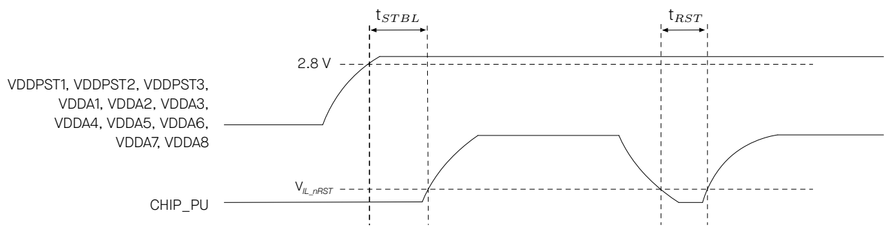
图 2-5. 上电和复位时序参数图
